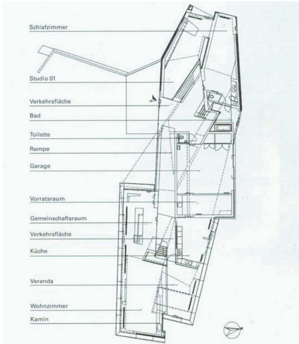
Geschossgrundriss Ebene 2 5
