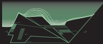
ERDGESCHOSS 1:100
